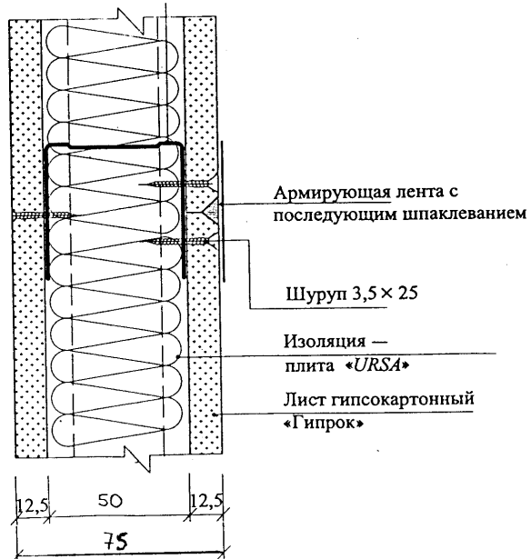
Рис. 2 Конструкция перегородки
